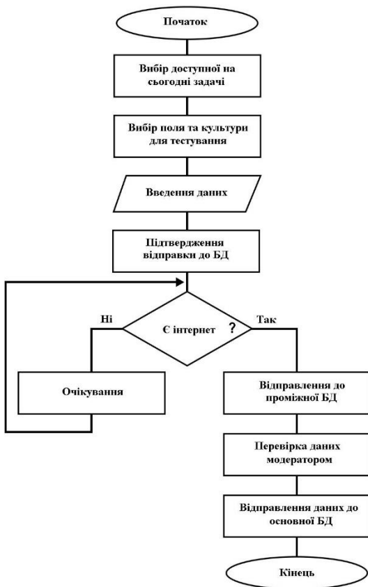
Рис. 1. Загальна блок-схема алгоритму функціонування програмного забезпечення мобільного додатку.
