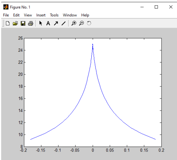
Рис. 2. Лістинг реалізації чисельного алгоритму побудови біфуркаційної множини для «Магічної формули» Н.В.Пасежка
