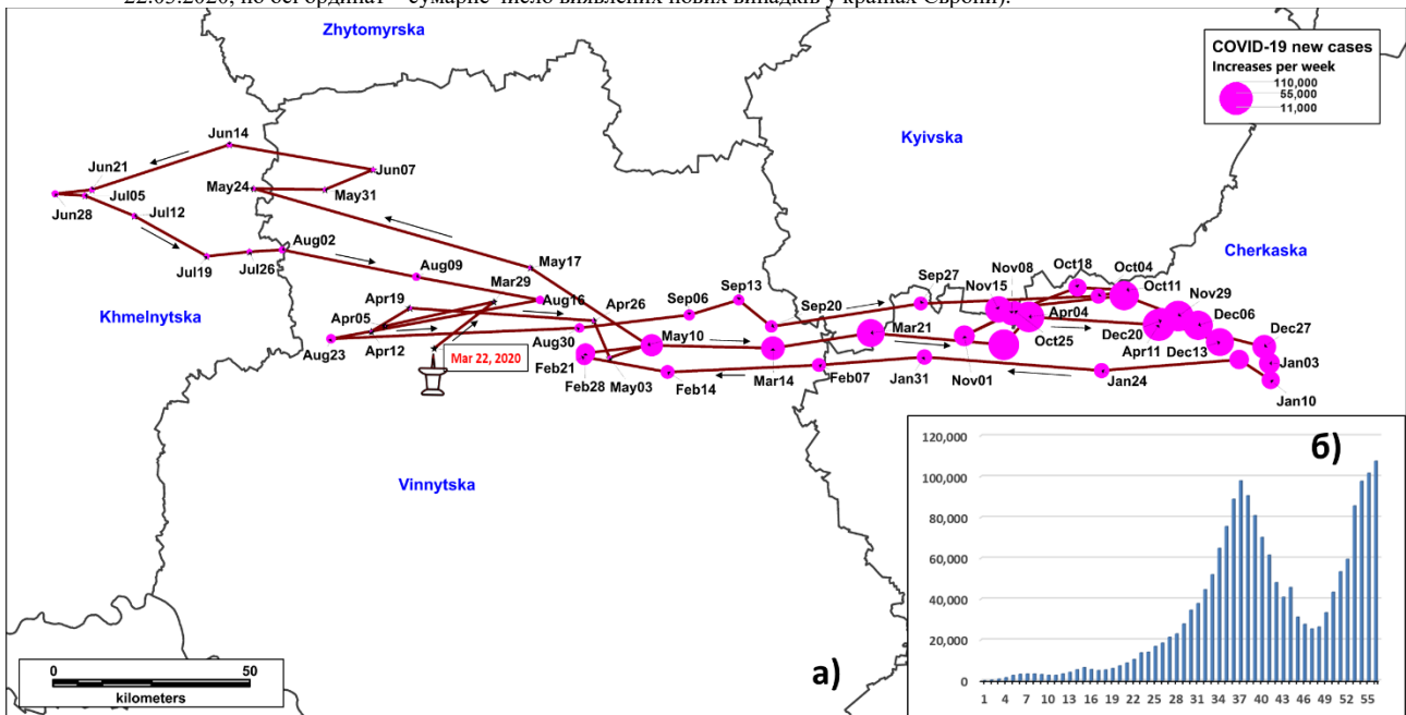
Рис. 3. Переміщення центру тяжіння для щотижневих нових випадків захворювання на COVID-9 в областях України: траєкторія центру тяжіння (а), починаючи з 22.03.2020, та піки захворюваності (б) (по осі абсцис – номери тижнів, починаючи з 22.03.2020, по осі ординат – число виявлених нових випадків).
