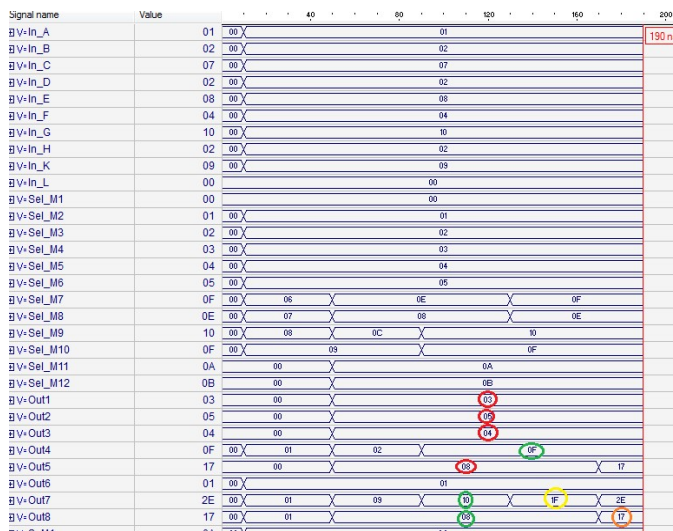
Рис. 4. Функціональна діаграма роботи реконфігуровного пристрою в середовищі Active-HDL.
