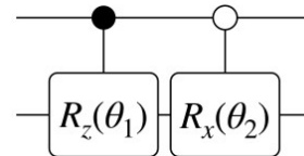
Рис. 4. Параметризована квантова схема, яка використовується в шарі пулінгу [4].
