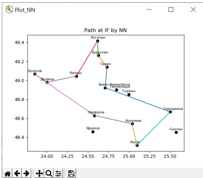
Рис. 3. Граф "Nearest_Neighbour".
