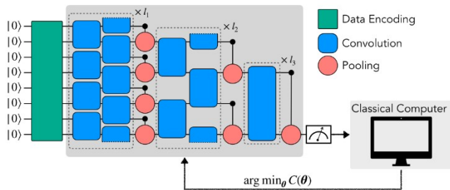
Рис. 1. Схематичне зображення квантової нейронної мережі [4].
